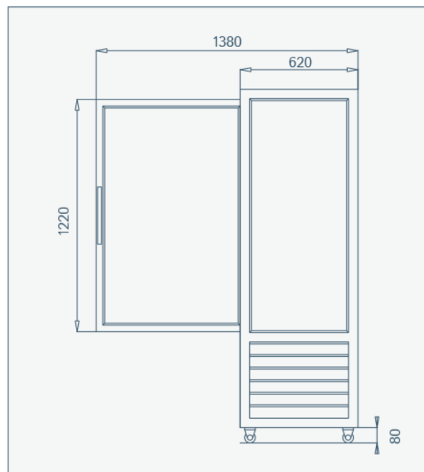
VISTA LATERALE
